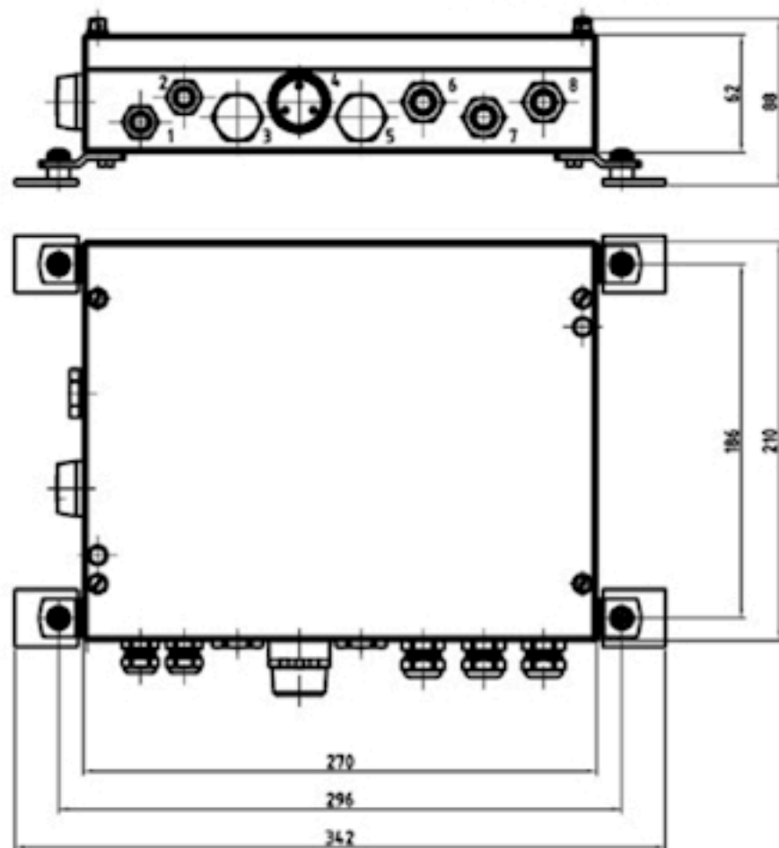
Zentraleinheit / central unit
